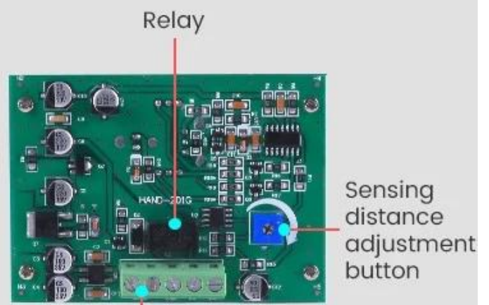
Wiring port
