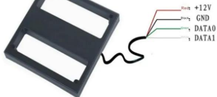
Wiring diagram(WG26 Format):
