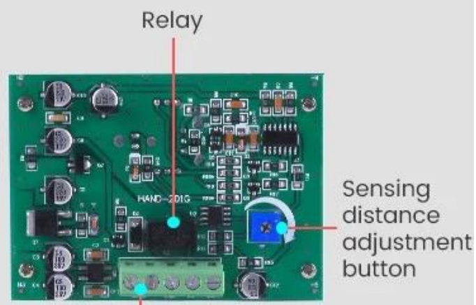
Wiring port
