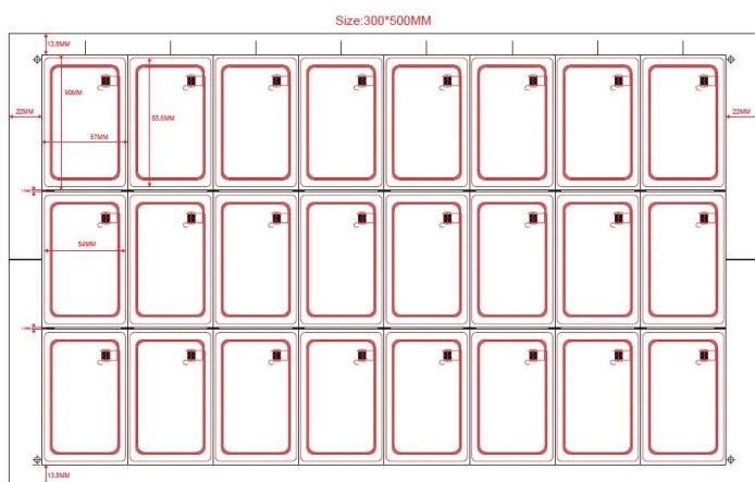
Layout 3x8
